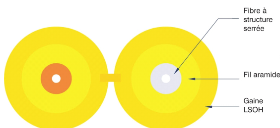
Coupe de profil du câble
