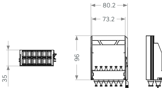
MD-12 Port MPO-Durchgangskassette
