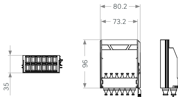
Cassette de passage MD-12 Port MPO
