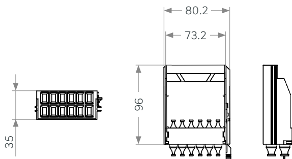
Kaseta przełotowa MD-12 Port MPO
